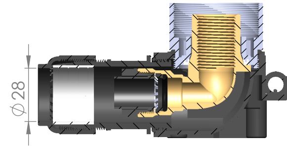
SECTION A-A SCALE 1 : 2
