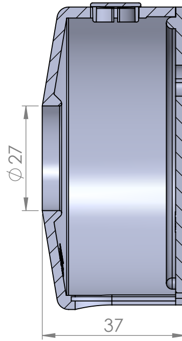
SECTION A-A
