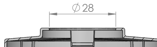
SECTION A-A
