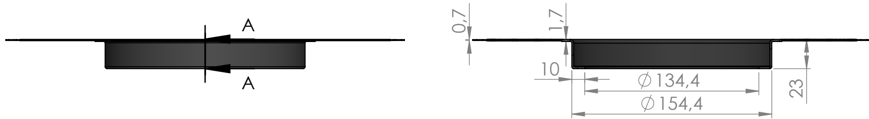
SECTION A-A SCALE 1 : 3
