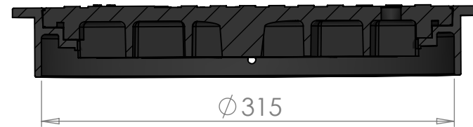
SECTION A-A SCALE 1 : 4
