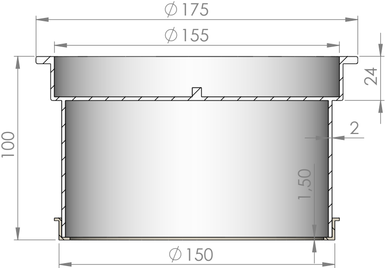
SECTION A-A SCALE 1 : 2
