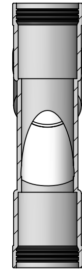
SECTION A-A SCALE 1 : 2
