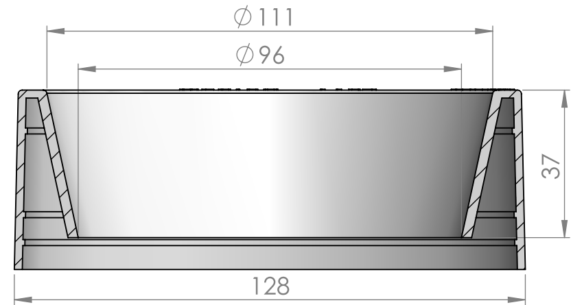
SECTION A-A SCALE 1 : 1.3
