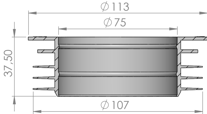
SECTION A-A SCALE 1 : 1.5
