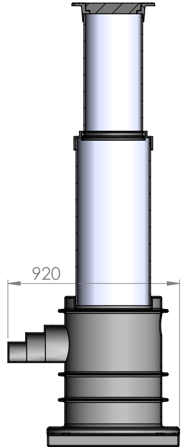
SECTION A-A SCALE 1 : 20
