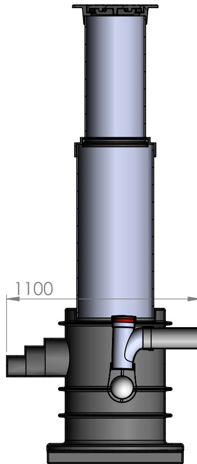
SECTION A-A SCALE 1 : 20
